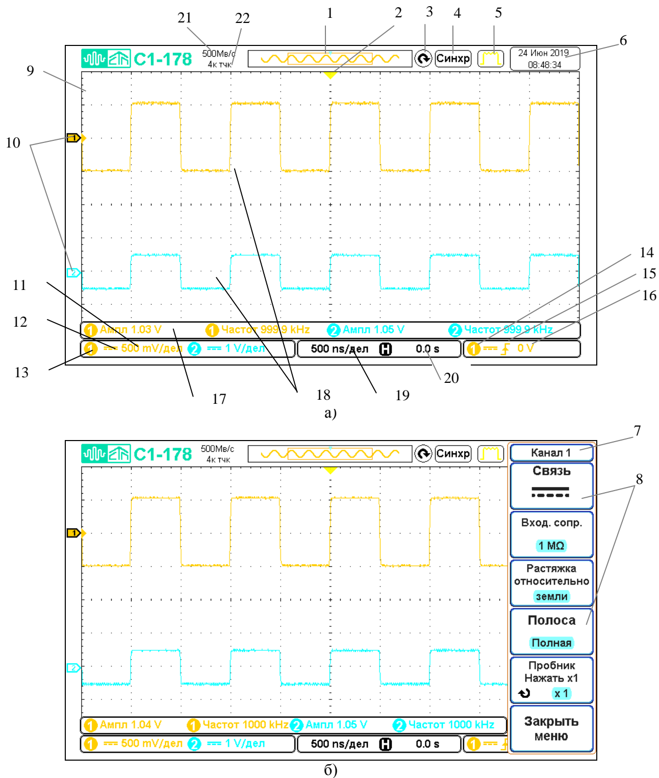
Рисунок 6.3 – Интерпретация показаний на экране осциллографа а) экранное меню выключено б) экранное меню включено
