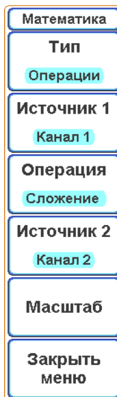
Рисунок 6.11 – Экранное меню «Математика» при выборе параметра «Тип/Операции»
