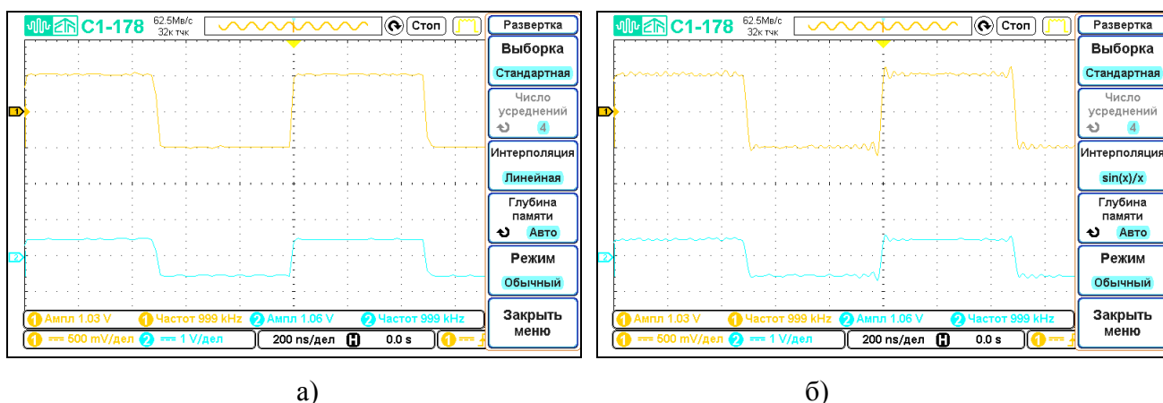
Рисунок 6.5 – Влияние режима интерполяции на отображаемую форму сигнала: а) линейная интерполяция б) интерполяция \sin(X)/X .
