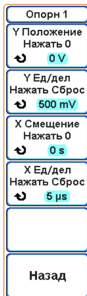
Рисунок 6.17 – Экранное меню «Опорн 1»
